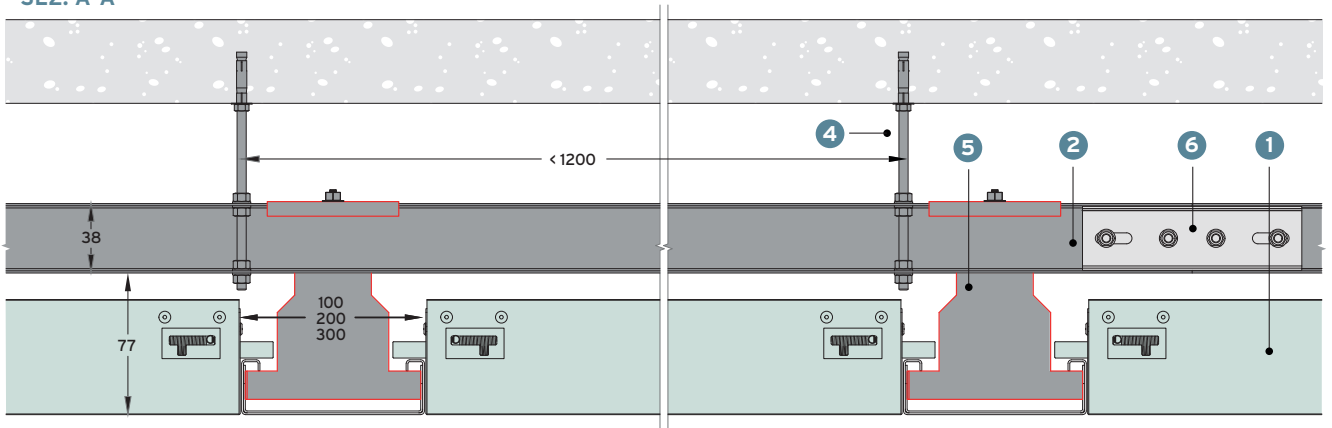
SEZ. A-A
