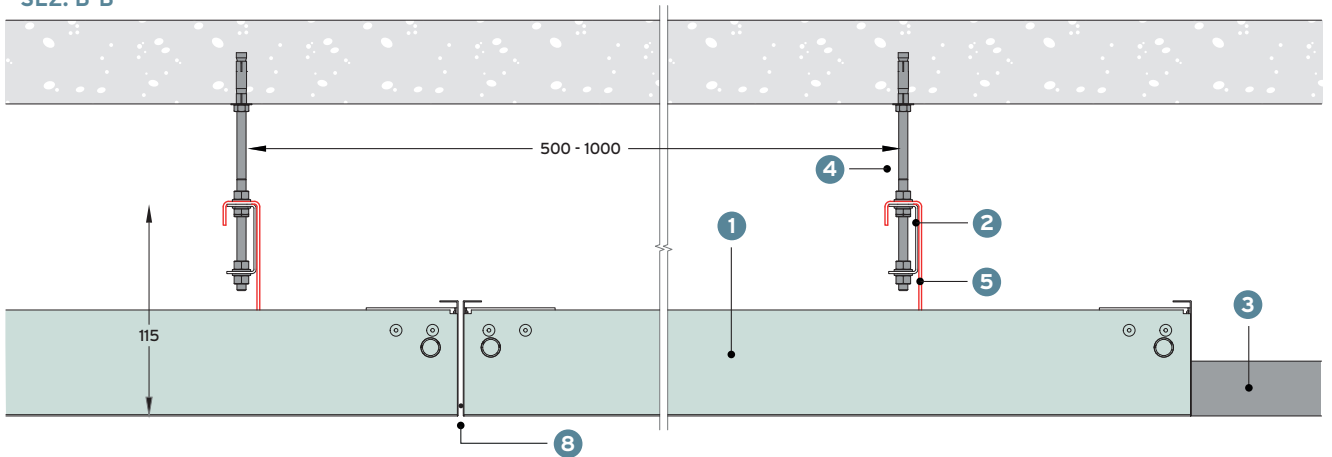
SEZ. B-B
