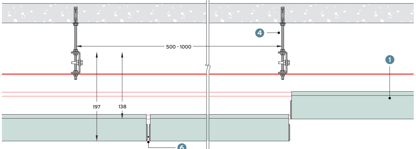
SEZ. B-B
